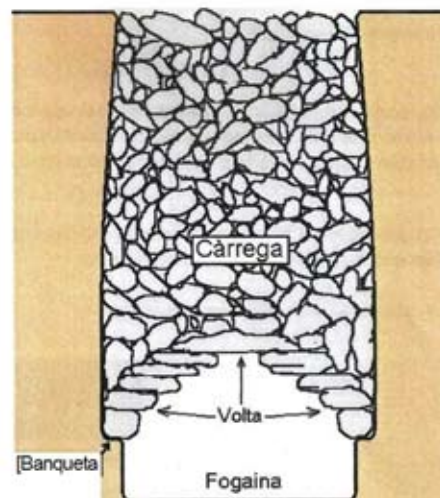
Secció d'un forn de guix
